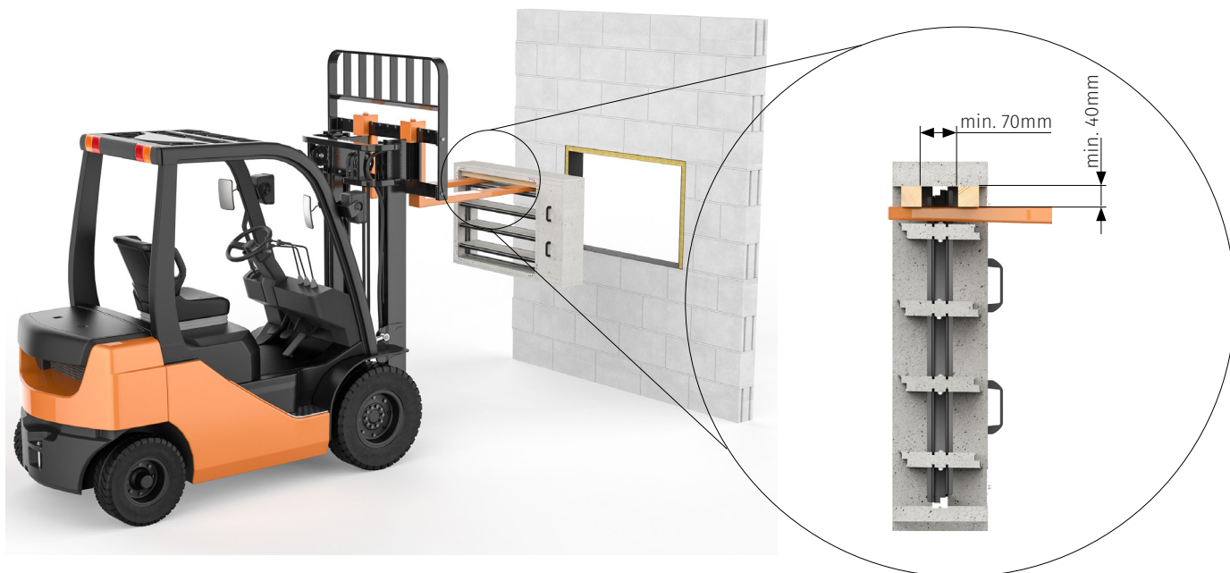
Detajl: leseni nosilci
